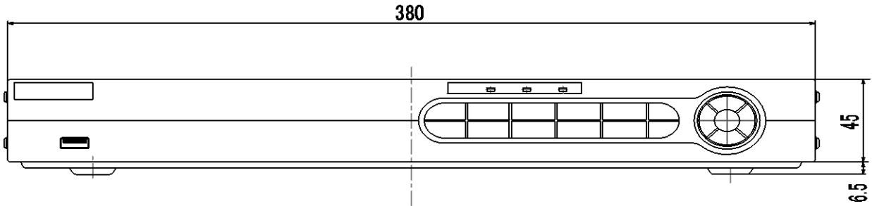
外形寸法図
